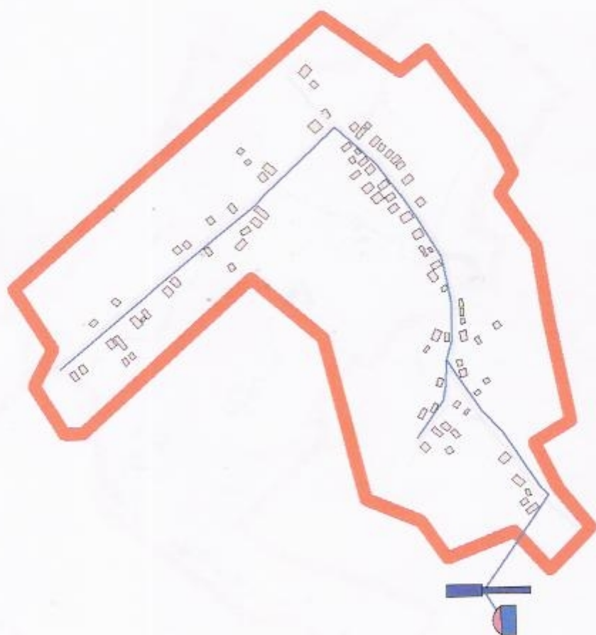
Рис 14 Водоснабжение Гартцевского сельского поселения Вязовск
