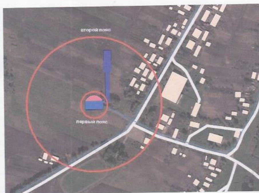
Рис.36 Зоны санитарной охраны ВЗУ2 Кобалево.
